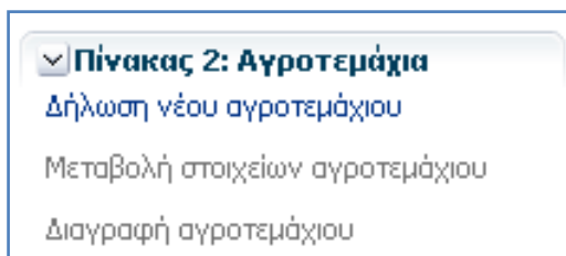
Εικόνα 32
